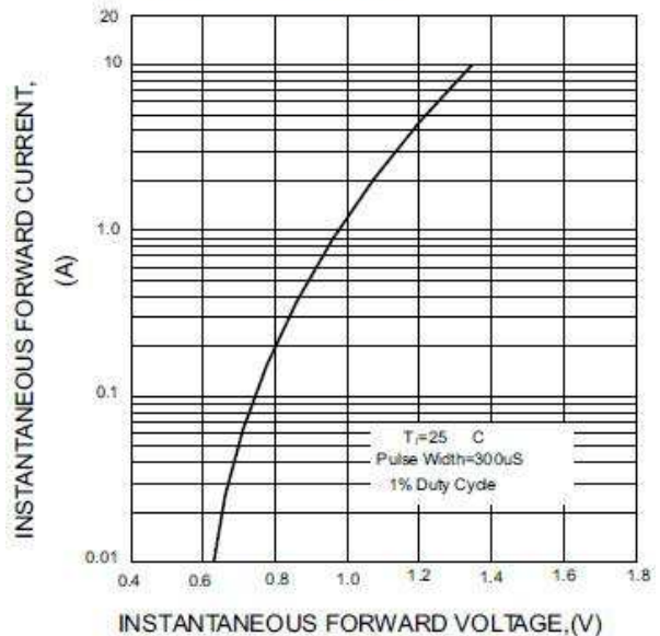
图4. 电性正向特性曲线
