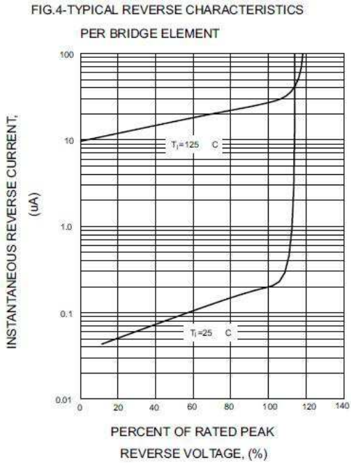
图5. 典型反向特性曲线
