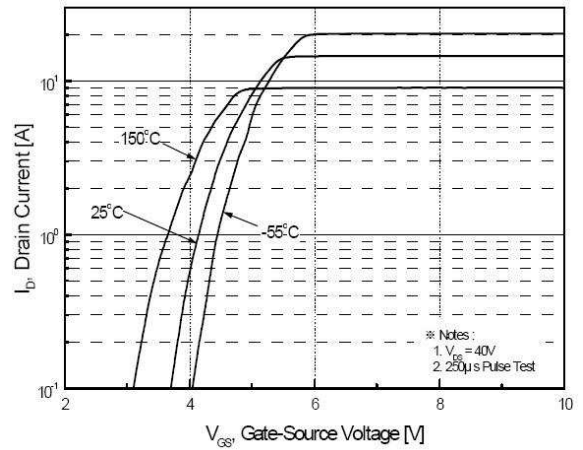
图2. 传输特性曲线
