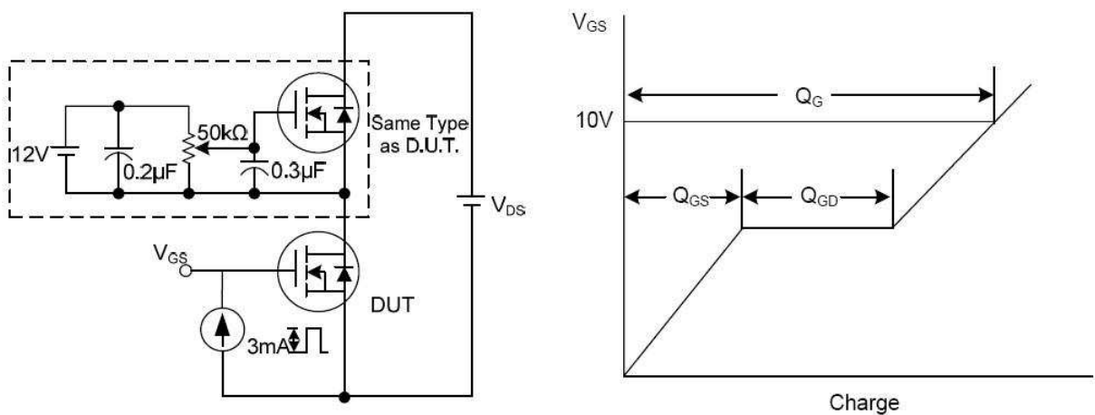
图12. 栅电荷测试
