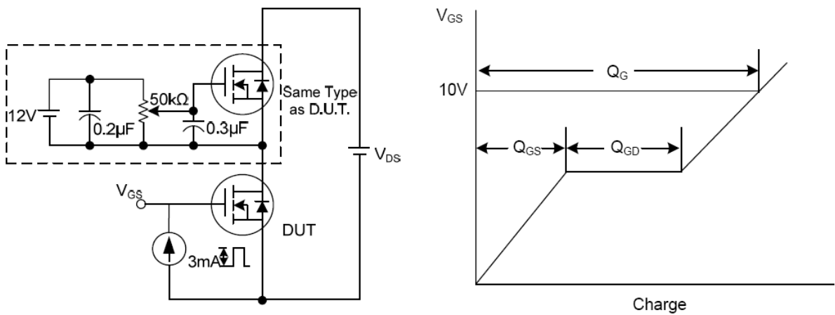
图12. 栅电荷测试
