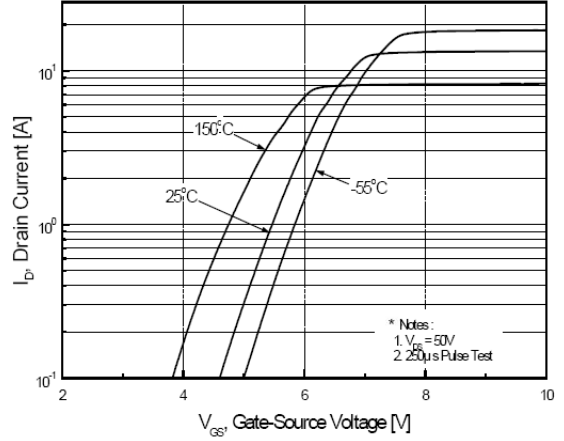
图2. 传输特性曲线 Fig. 2 Transfer Characteristics
